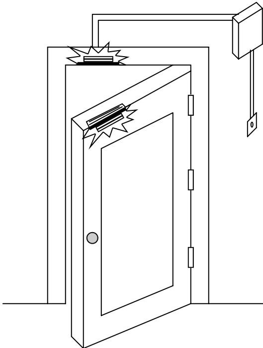
ROFU 8035 Mini Shear Lock Mortise Installation
